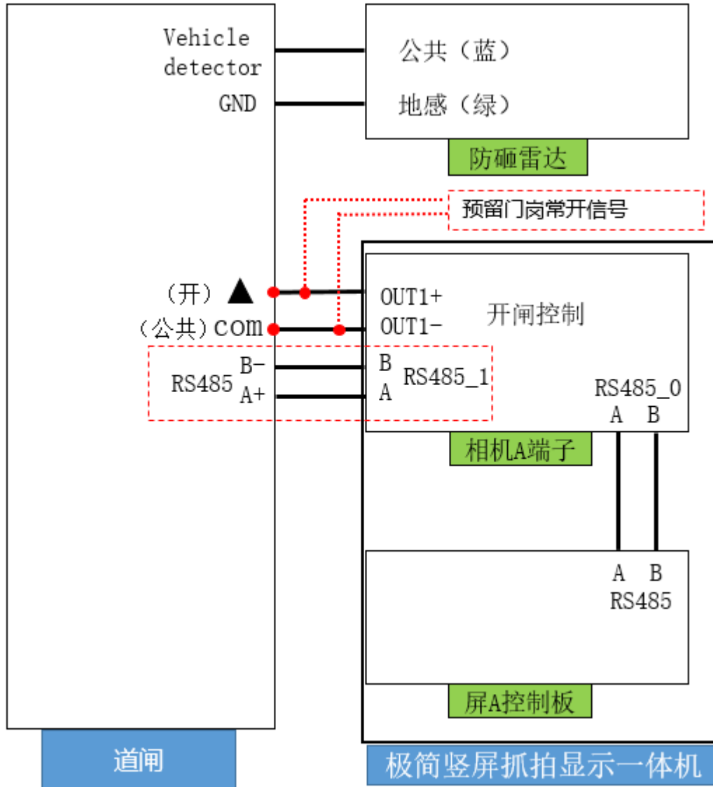
图4-2 整体接线示意图
