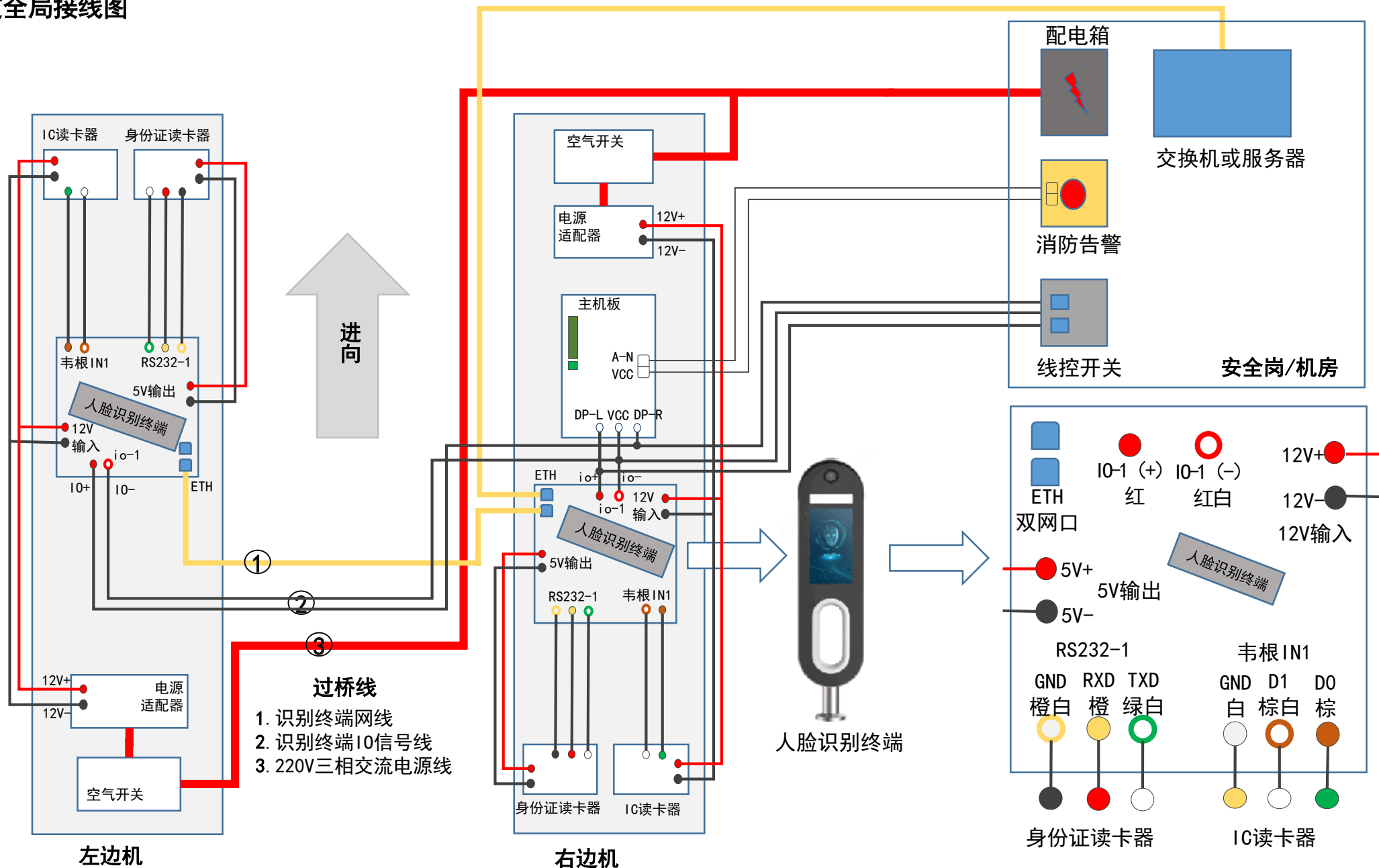
人脸识别终端接线图
