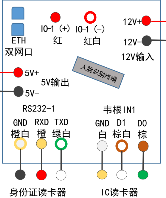
人脸识别终端接线图
