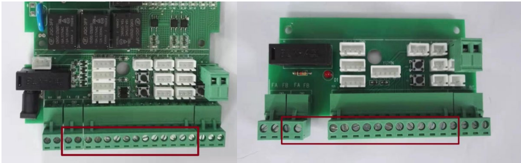
图7-7 DEL 系列速通门主机板与辅机板过桥线示意图
