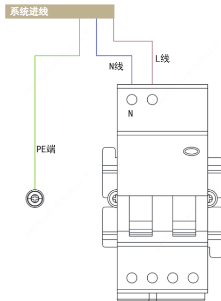
图7-1 速通门电源空开接线示意图
