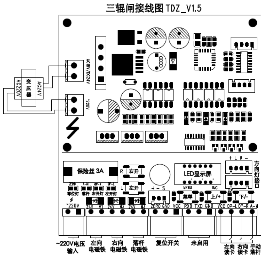
图7-3 DEL-511 系列三辊式速通门主板接线图
