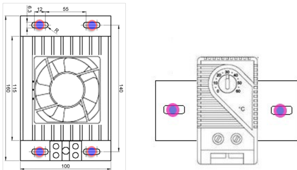
图8-4 固定安装示意图
