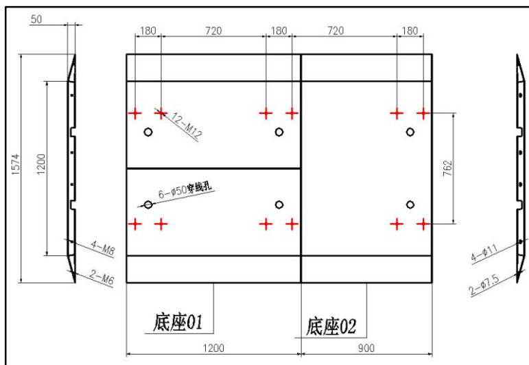
图8-6 DEL 系列速通门底座 01+底座 02 组合规格
