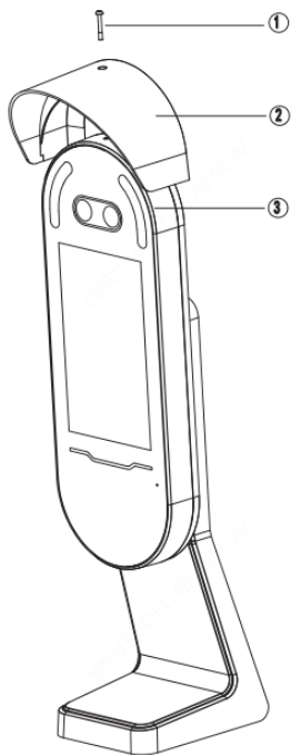
图1-8 遮阳罩安装示意图
