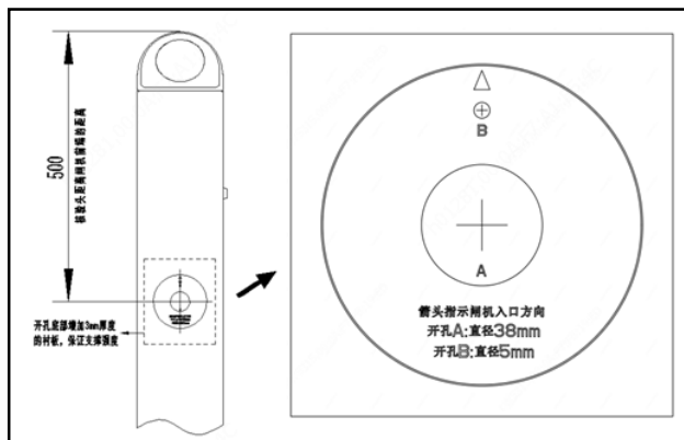
图1-1 人脸速通门盖板开孔图
