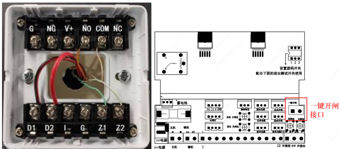
图8-5 接线实物图
