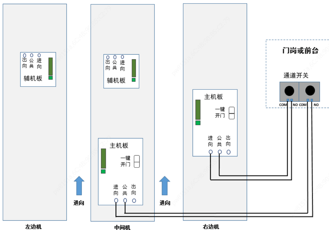
图8-2 通道开关接线示意图
