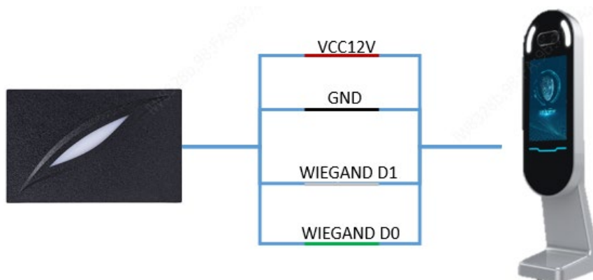
图1-8 人脸核验终端与 IC 读卡器接线图
