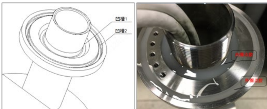
图1-3 识别终端点胶图
