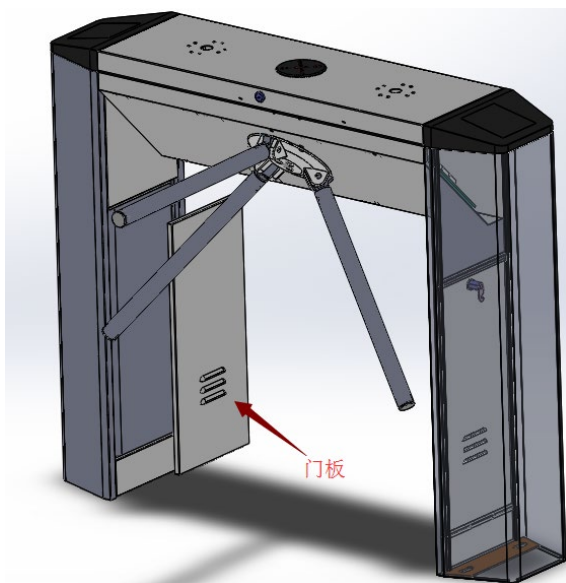
图6-3 速通门部分拆卸图
