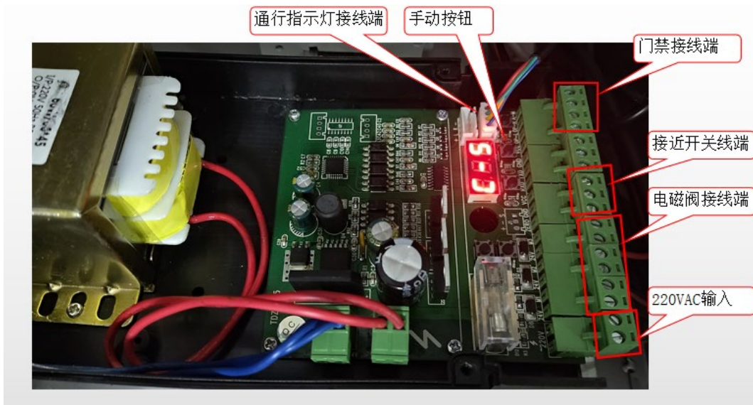
图7-3 DEL-511 系列三辊式速通门主板接线图
