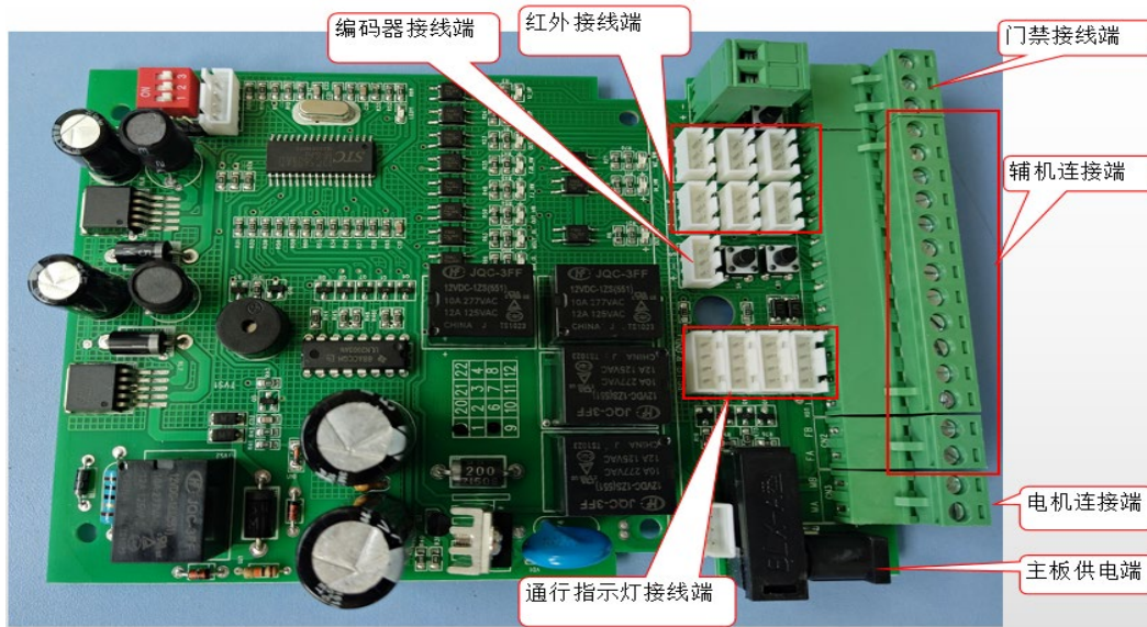
图7-4 DEL-611 翼式速通门主控板接线图
