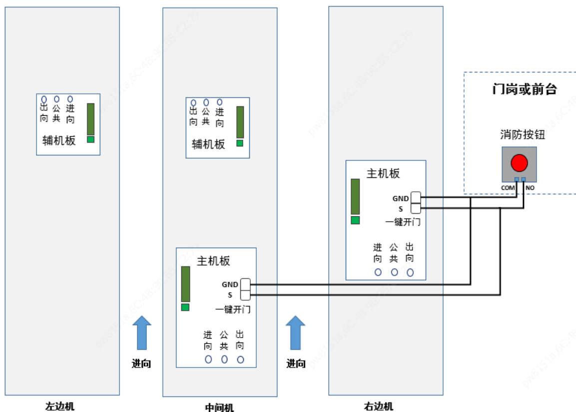
图8-1 消防按钮接线示意图
