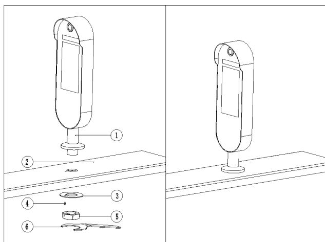
图1-7 人脸识别终端安装图
