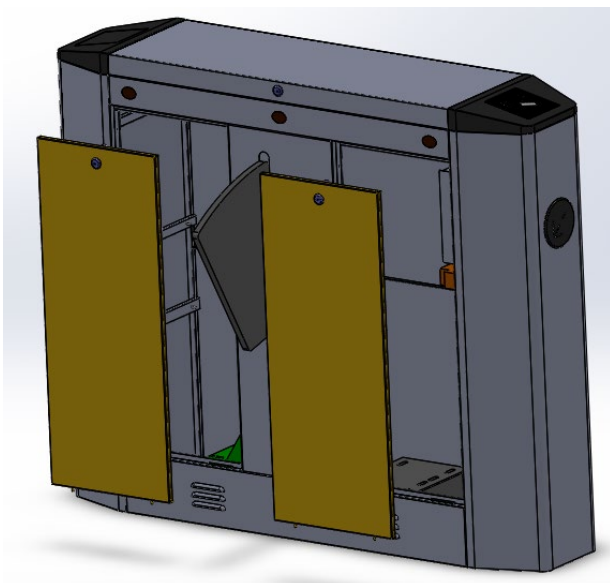
图6-6 速通门部分拆卸图
