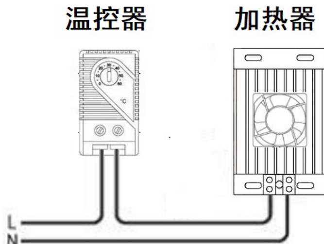
图8-3 温控模块接线方式
