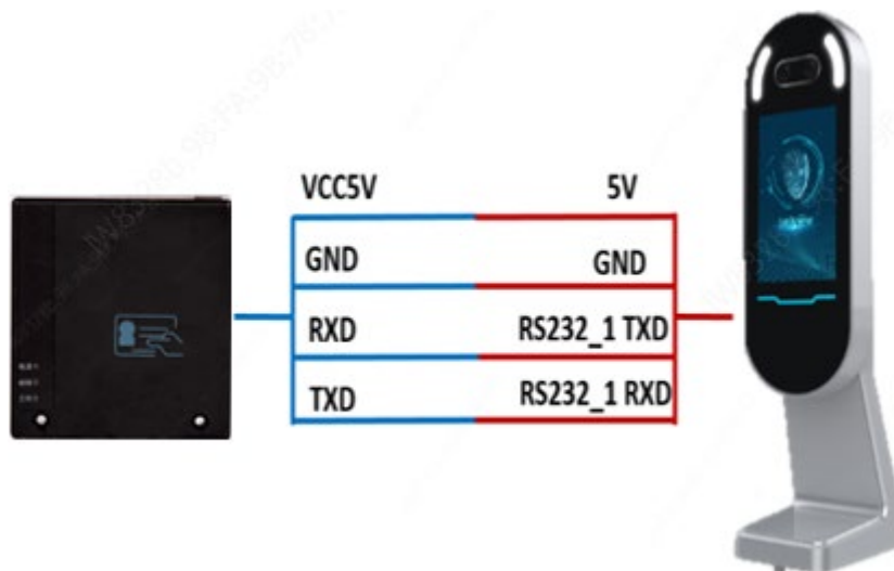
图7-10 人脸识别终端与身份证读卡器接线图
