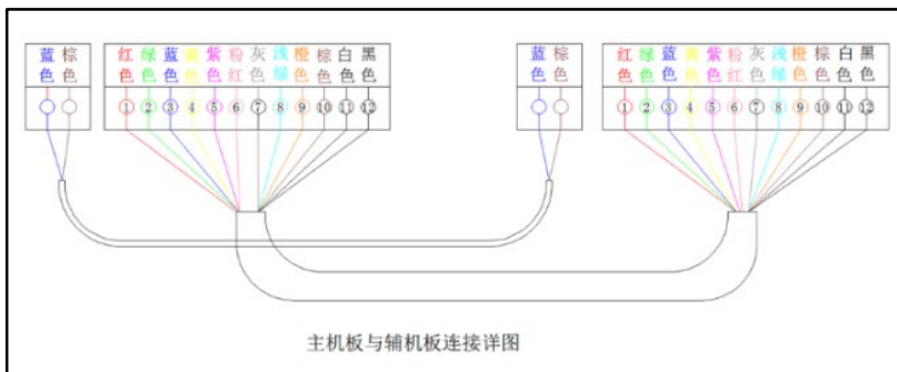
图7-7 DEL 系列速通门主机板与辅机板过桥线示意图
