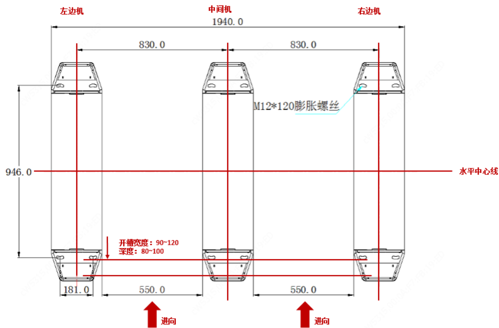
图6-2 通道安装尺寸图
