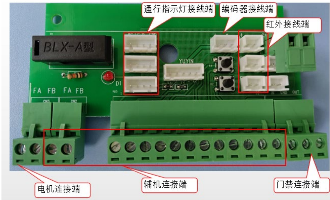
图7-5 DEL-611 翼式速通门通道副机接线图
