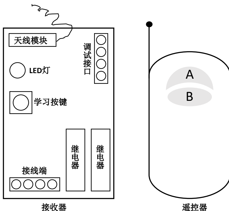
图 8-3 接收板/遥控器
