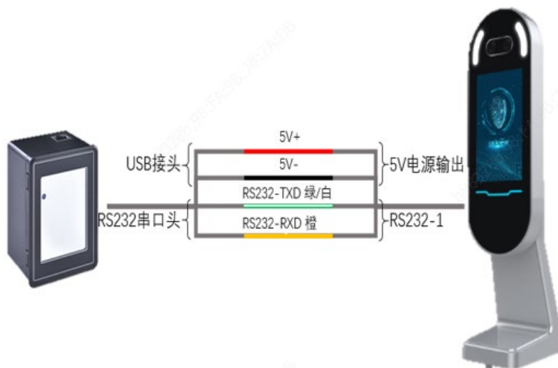
图7-12 二维码读卡器接线图
