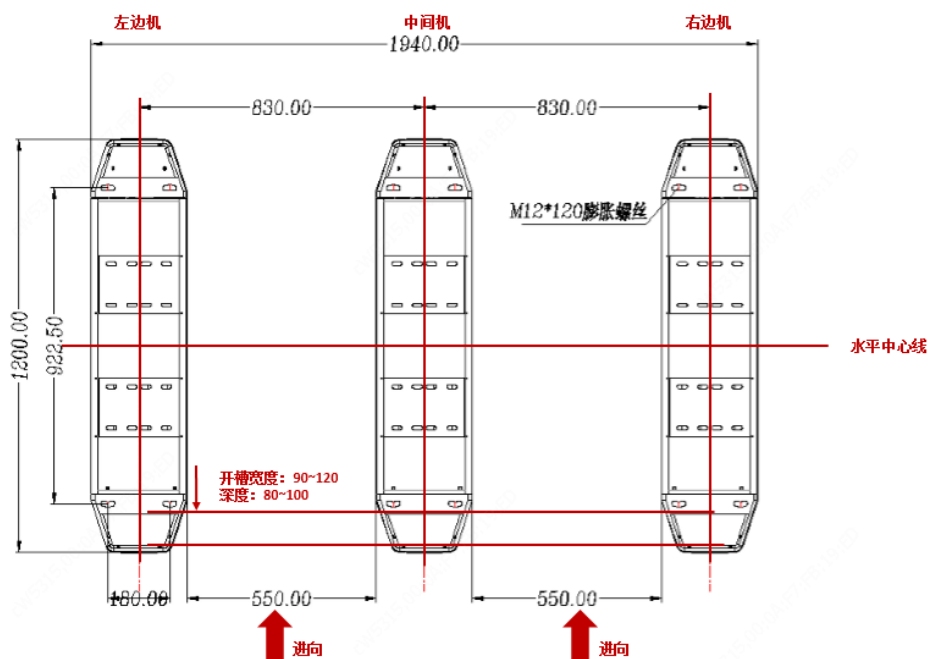
图6-5 通道安装尺寸图（底视图）
