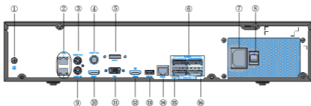
图2-1 示例设备 1
