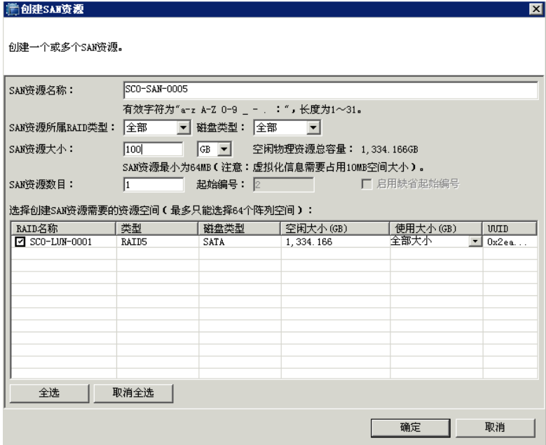
图3-6 创建逻辑资源
