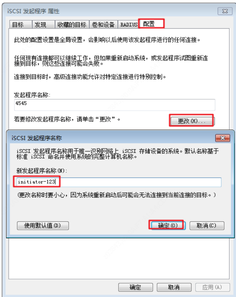
图3-12 设置 initiator 名称
