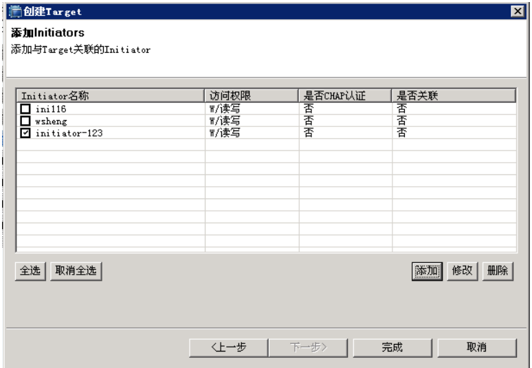
图3-10 设置 Target 和 Initiator 关联
