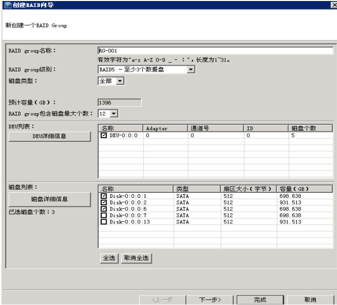
图3-3 创建 RAID Group
